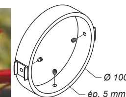
559 Décor Ø100 mm Aluminium laqué
