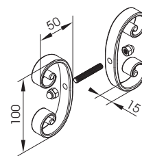
663 Paire de volutes intermédiaires Aluminium
