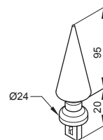
667 Embout flèche Aluminium
