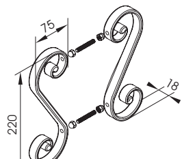
664 Paire de volutes centrales Aluminium
