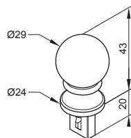
666 Embout boule Aluminium
