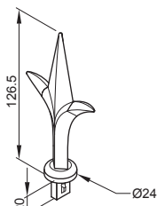
665 Embout fleur de lys Aluminium
